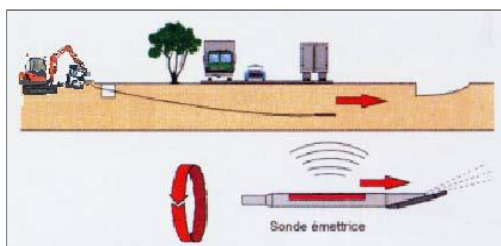
1 - La réalisation du tir pilote.
